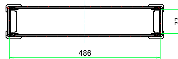
A-A ( 1 : 7.5 )
