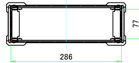
A-A (1:6)
