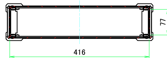
A-A ( 1 : 6.5 )
