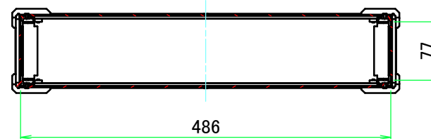
A-A (1:7)
