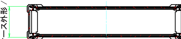
D-D (1:7)
