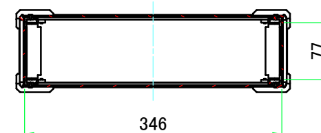
A-A (1:7)
