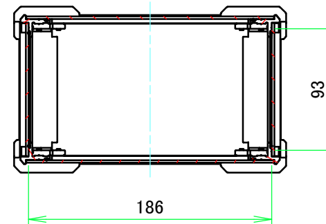
A-A (1:4)
