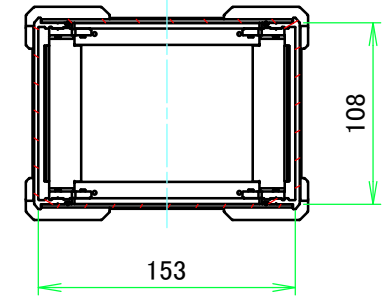
C-C ( 1 : 4.5 )
