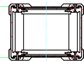
D-D (1:5)
