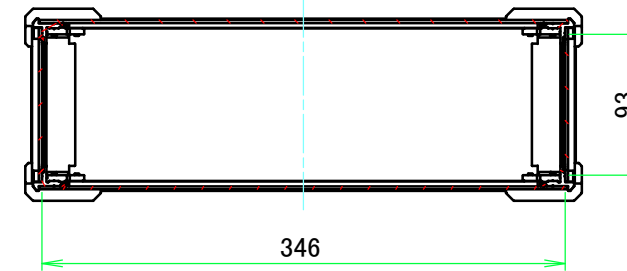
A-A (1:5)
