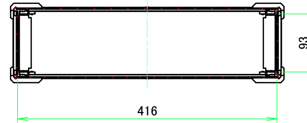
A-A (1:6)
