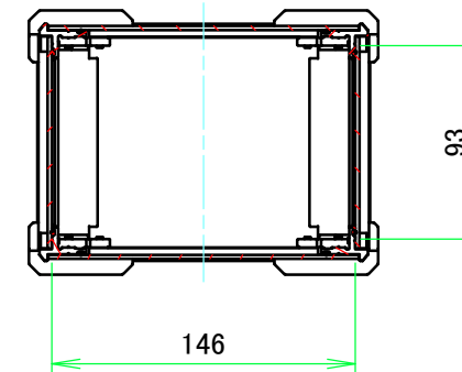
A-A (1:4)
