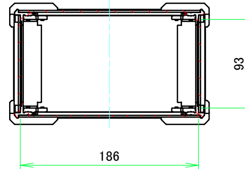
A-A (1:4)
