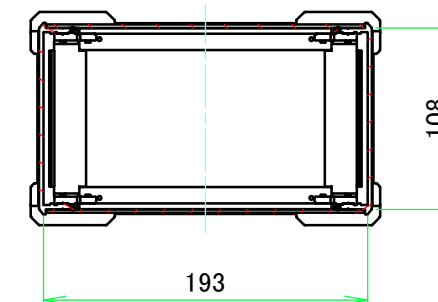
C-C ( 1 : 4.5 )
