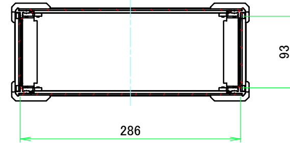
A-A (1:5)
