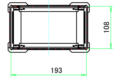
C-C ( 1 : 5.5 )
