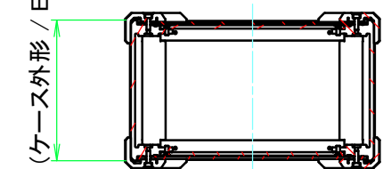
D-D ( 1 : 5.5 )
