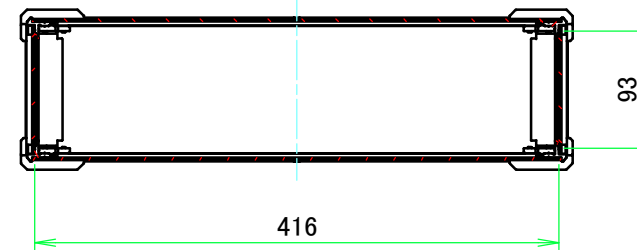
A-A (1:6)
