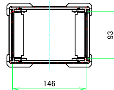
A-A ( 1 : 4.5 )
