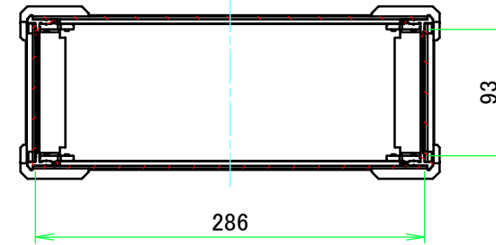
A-A (1:5)
