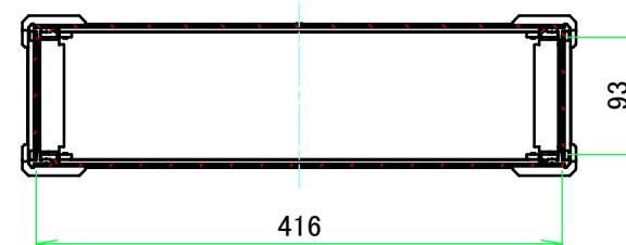
A-A (1:6.5)
