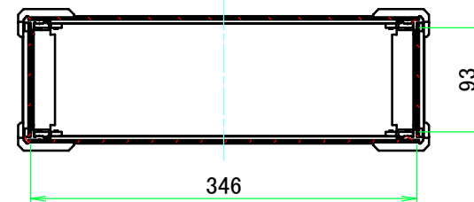
A-A (1:6)
