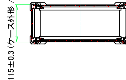
D-D (1:7)
