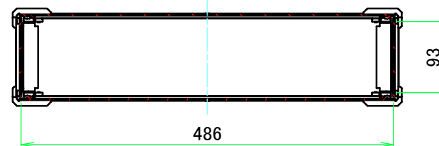
A-A (1:7)
