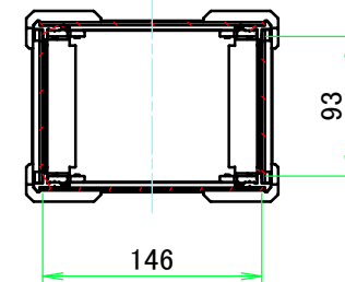
A-A ( 1 : 5.5 )
