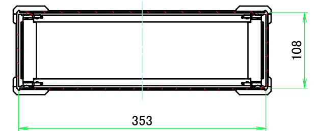
C-C ( 1 : 5.5 )
