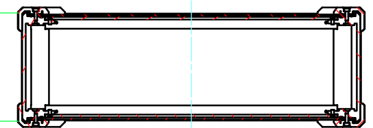
D-D ( 1 : 5.5 )
