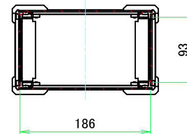
A-A ( 1 : 5.5 )
