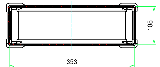
C-C ( 1 : 5.5 )
