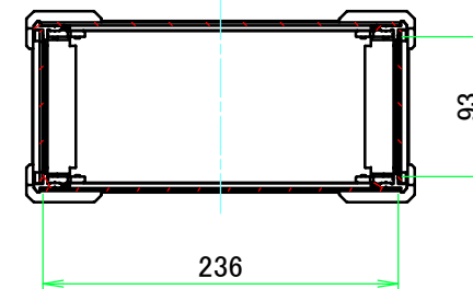
A-A ( 1 : 5.5 )
