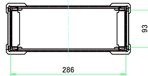
A-A ( 1 : 5.5 )
