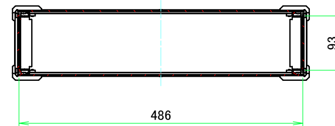
A-A (1:6.5)
