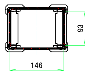
A-A (1:6)
