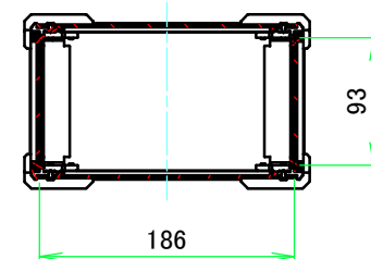
A-A (1:6)
