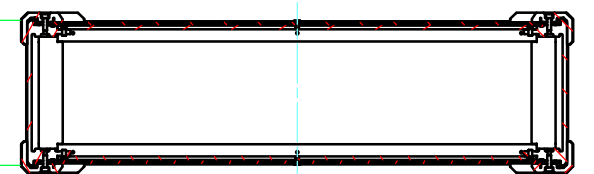
D-D (1:6)
