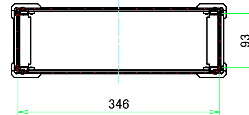
A-A (1:6.5)
