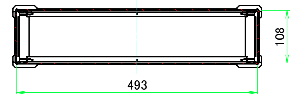
C-C ( 1 : 7.5 )
