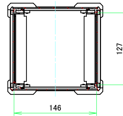
A-A (1:4)
