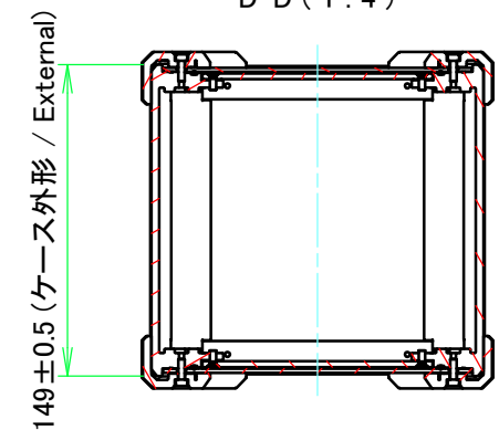
D-D (1:4)
