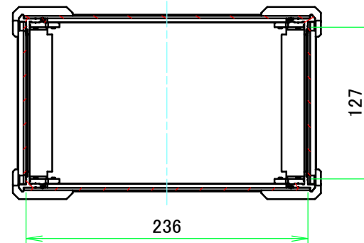
A-A ( 1 : 4.5 )
