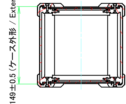
D-D ( 1 : 4.5 )
