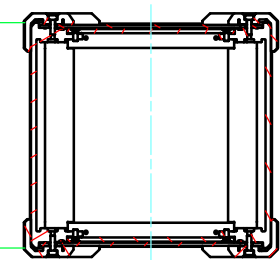
D-D (1:5)
