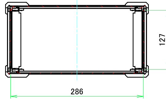
A-A (1:5)
