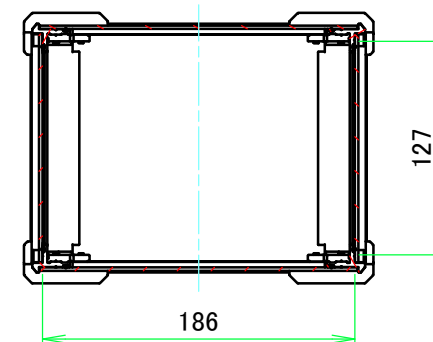
A-A ( 1 : 4.5 )
