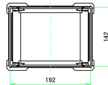
C-C ( 1 : 4.5 )
