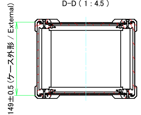
D-D ( 1 : 4.5 )
