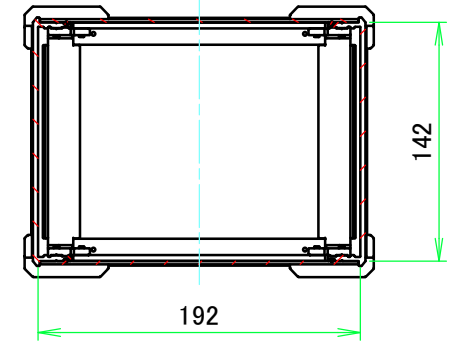
C-C ( 1 : 4.5 )
