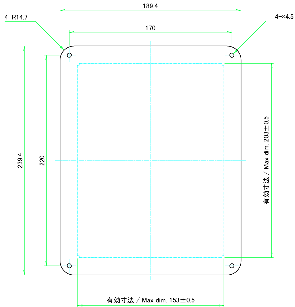
保護シート側 Surface protective film side
