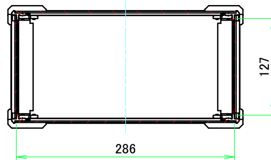
A-A (1:5)
