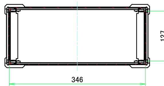
A-A ( 1 : 5.5 )
