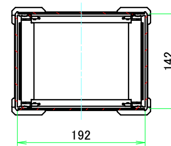
C-C ( 1 : 5.5 )
