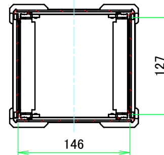
A-A (1:5)
