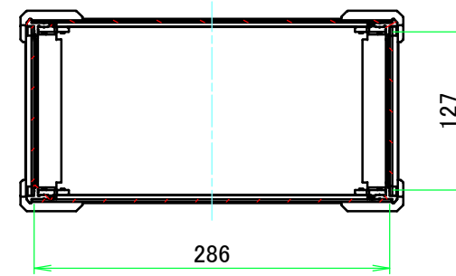
A-A ( 1 : 5.5 )
