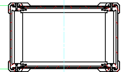
D-D ( 1 : 5.5 )
