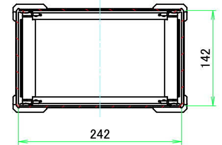
C-C ( 1 : 5.5 )
