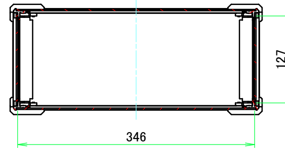
A-A ( 1 : 5.5 )
