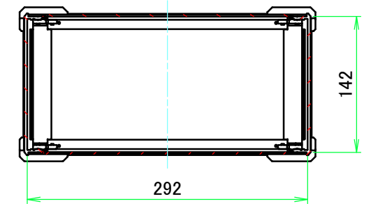
C-C ( 1 : 5.5 )
