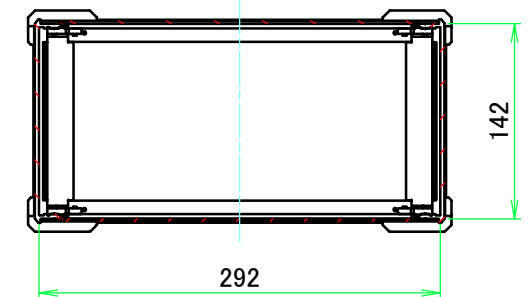
C-C ( 1 : 5.5 )
