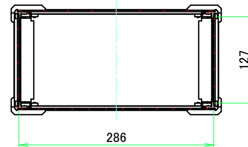
A-A ( 1 : 5.5 )
