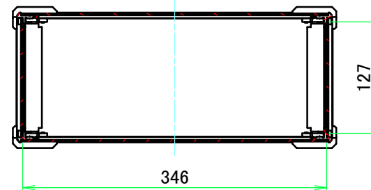
A-A (1:6)
