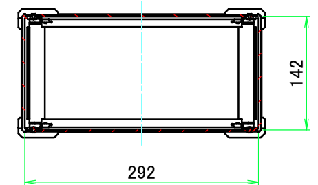
C-C ( 1 : 6.5 )
