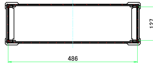
A-A (1:7)
