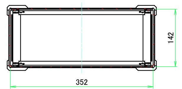
C-C ( 1 : 5.5 )
