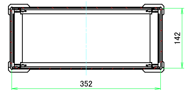
C-C ( 1 : 5.5 )
