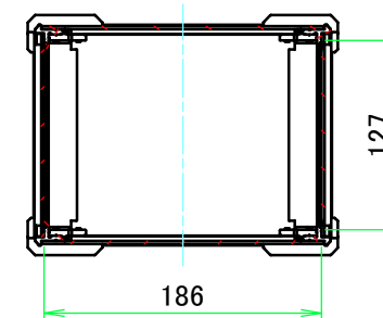
A-A ( 1 : 5.5 )
