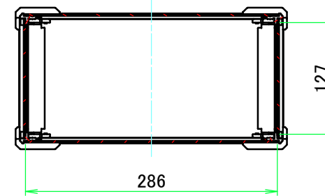
A-A (1:6)
